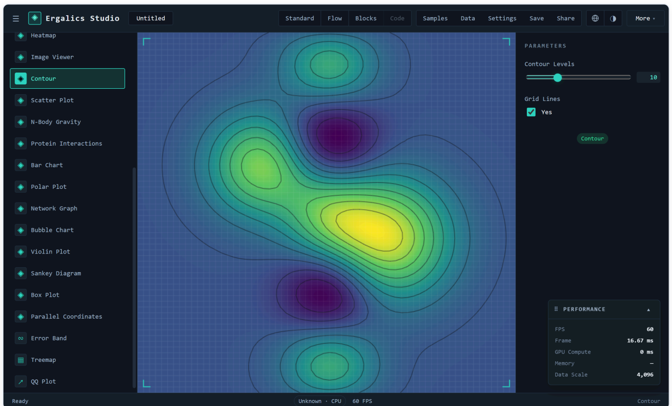
等值线：双高斯标量场
